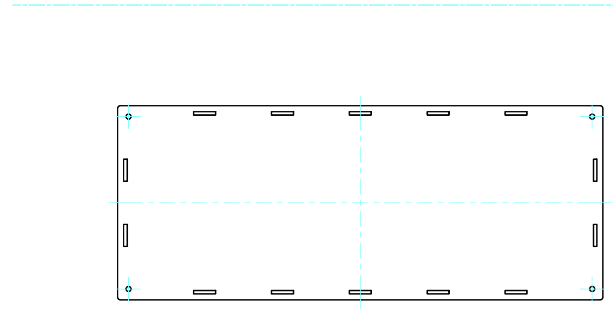
上カバー表面 / Top cover Frontside
