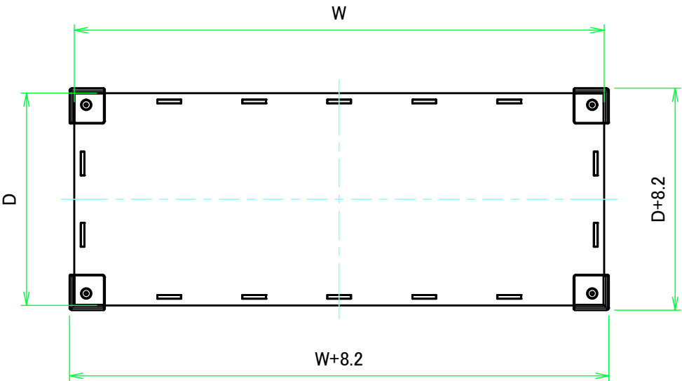
上カバー / Top cover
